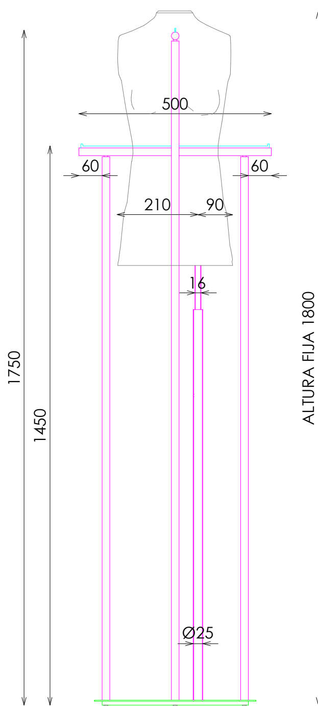
ALZADO FRONTAL
