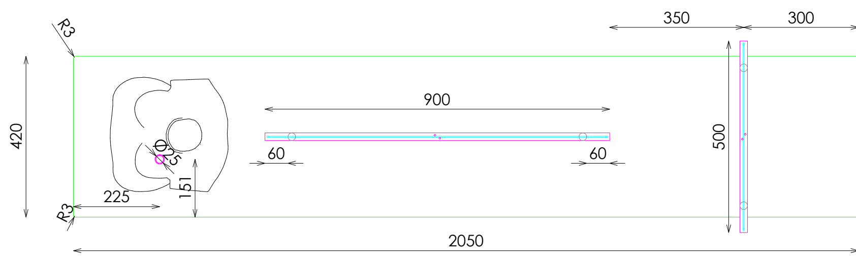
PLANTA
