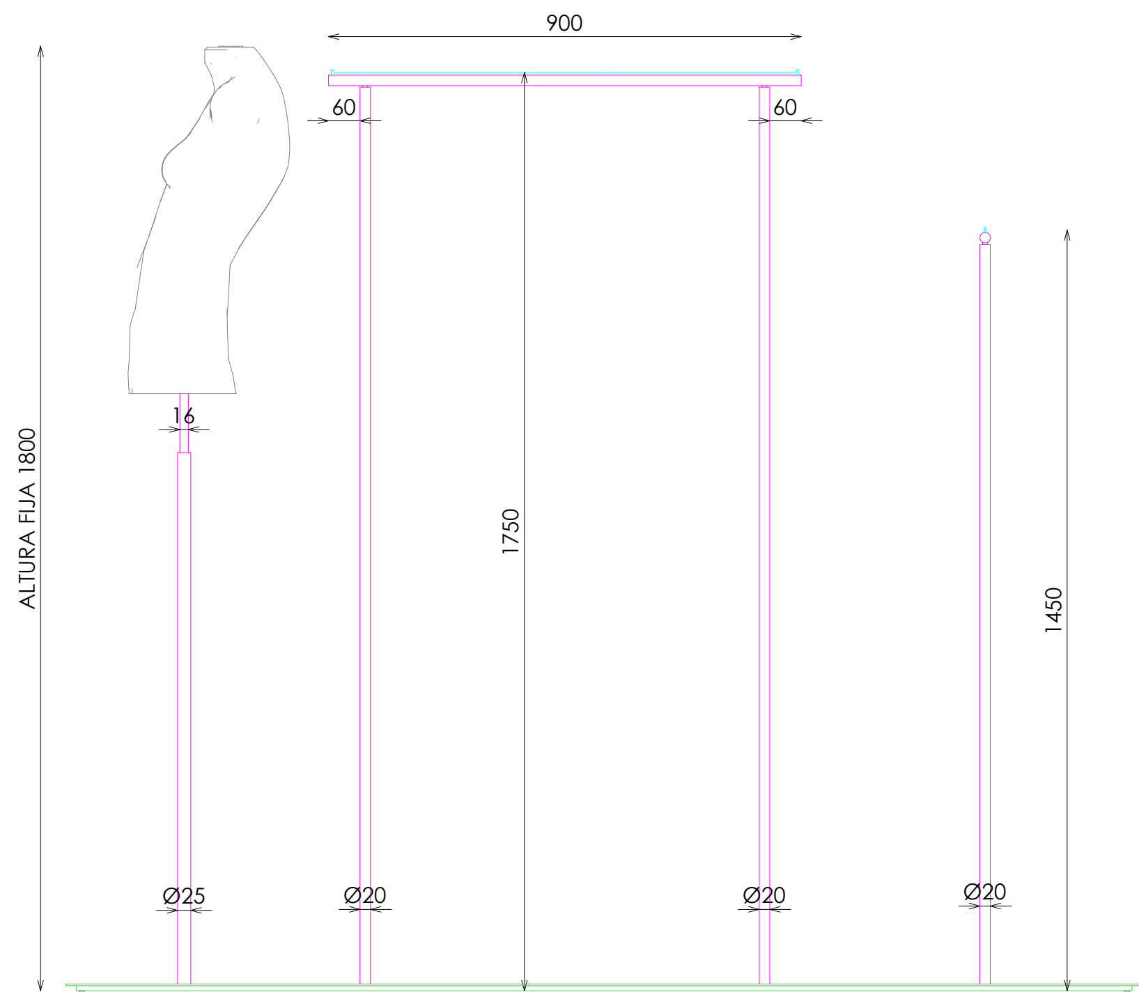
ALZADO LATERAL
