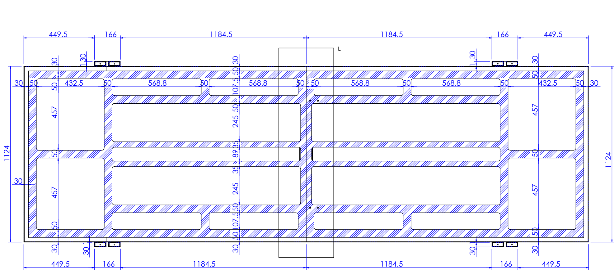
剖面 C-C
