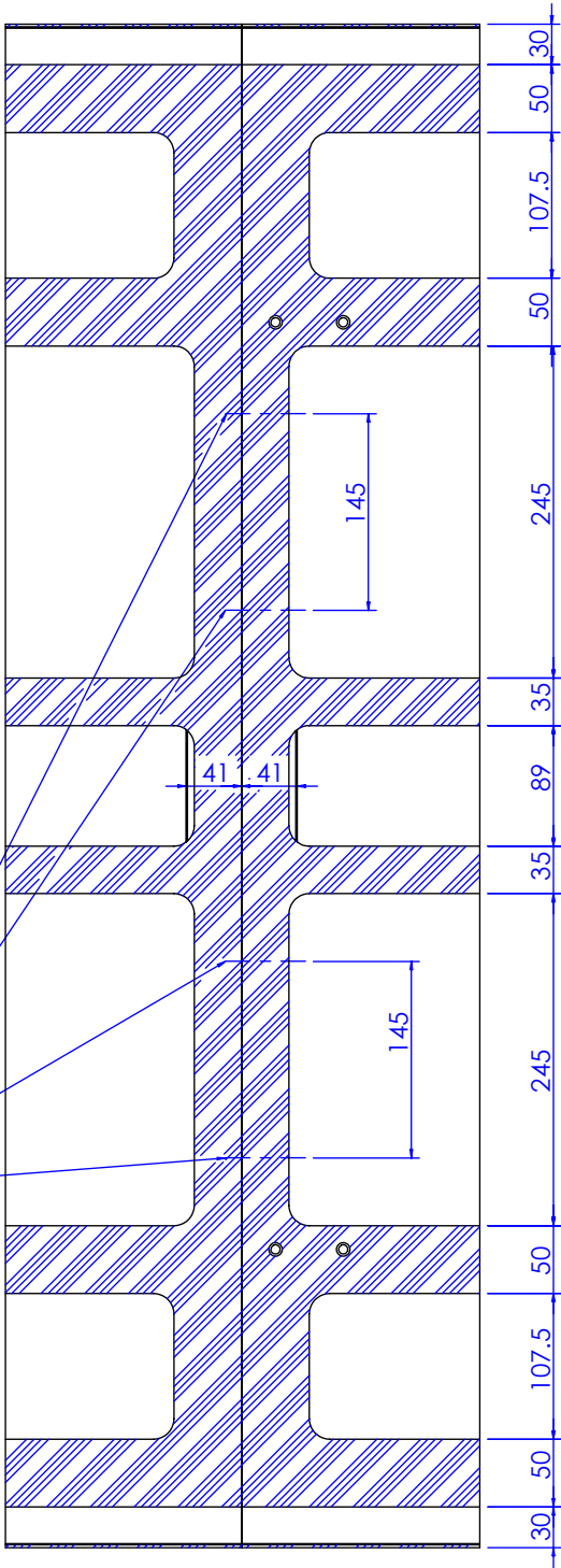
局部视图 L 比例 1:6
