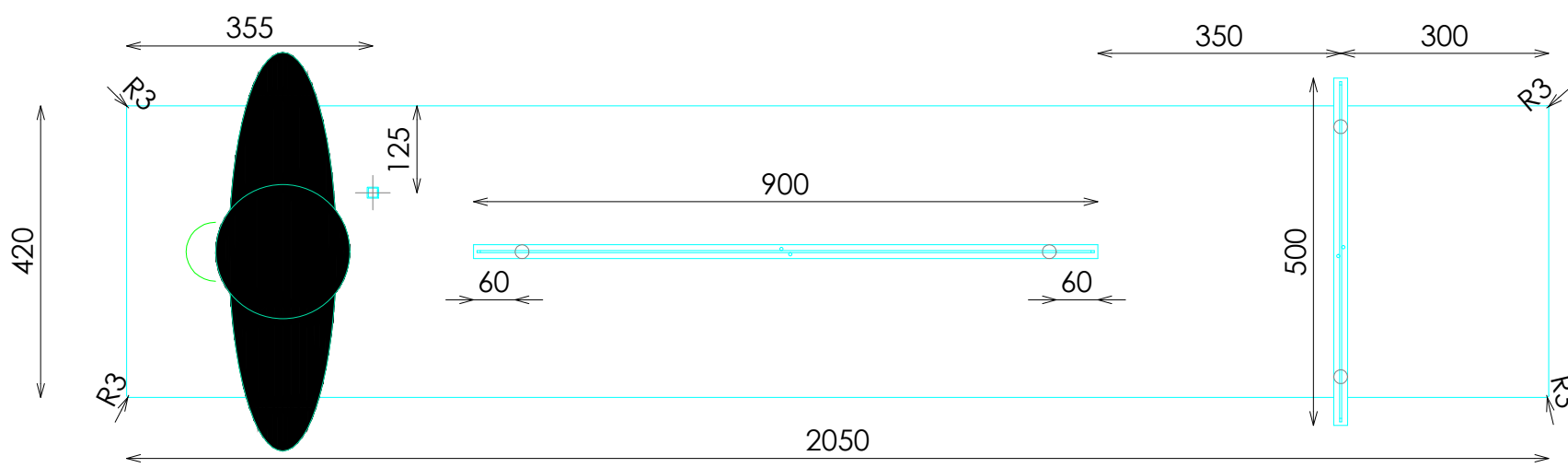
PLANTA
