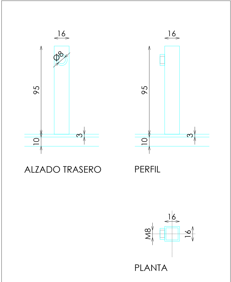
DETALLE ANCLAJE MANIQUI
