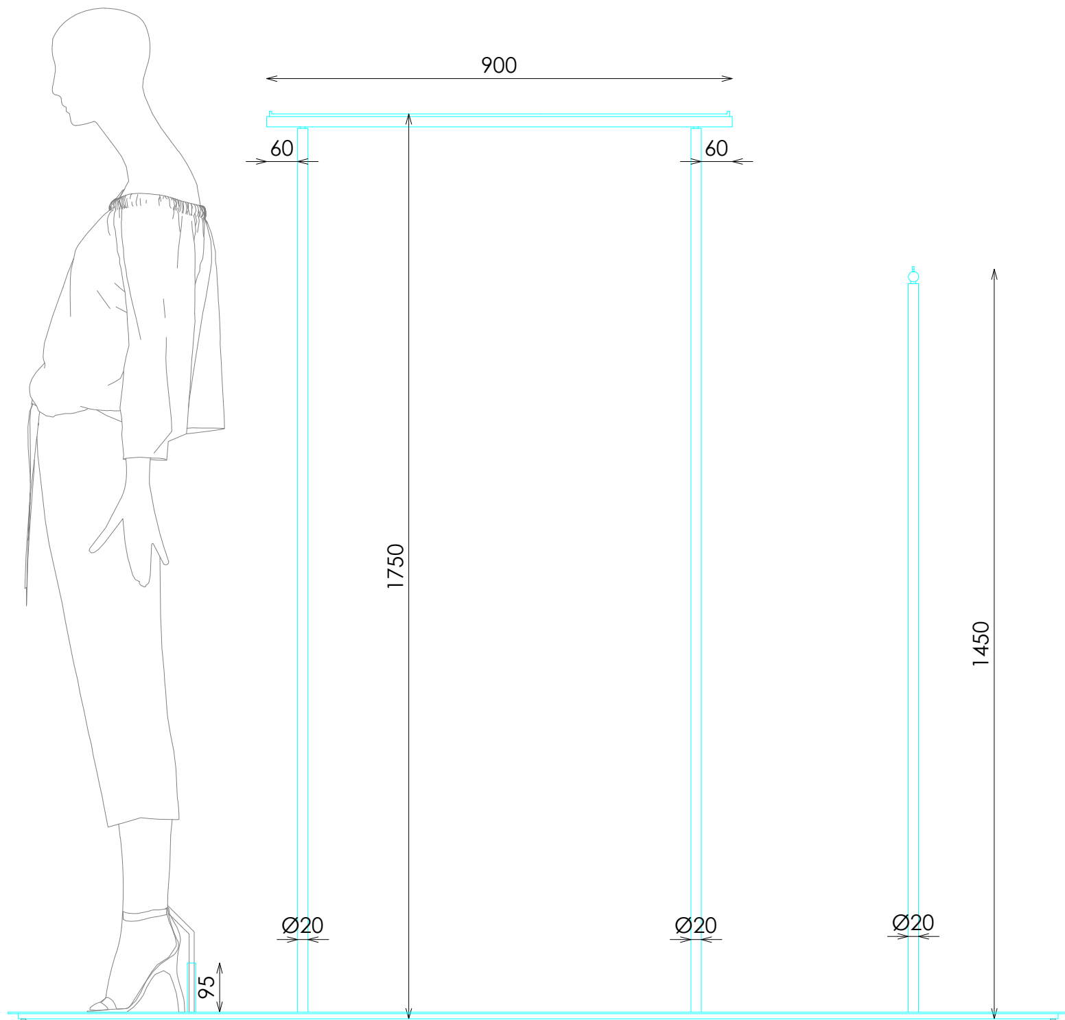
ALZADO LATERAL
