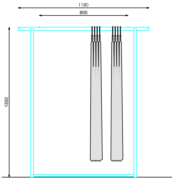
ALZADO
