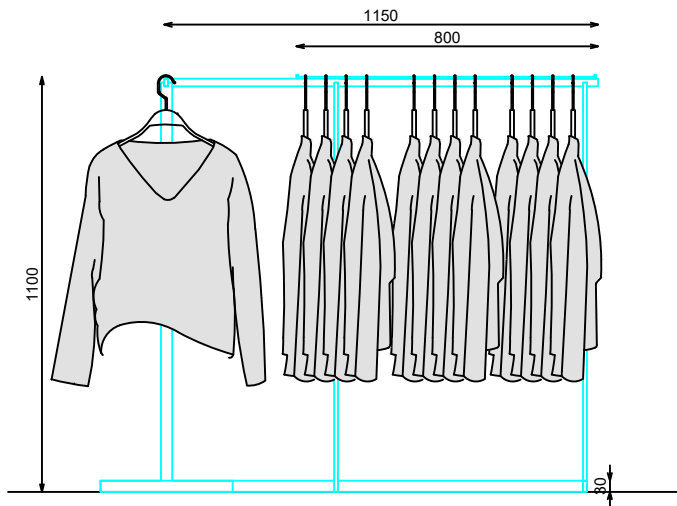
ALZADO FRONTAL
