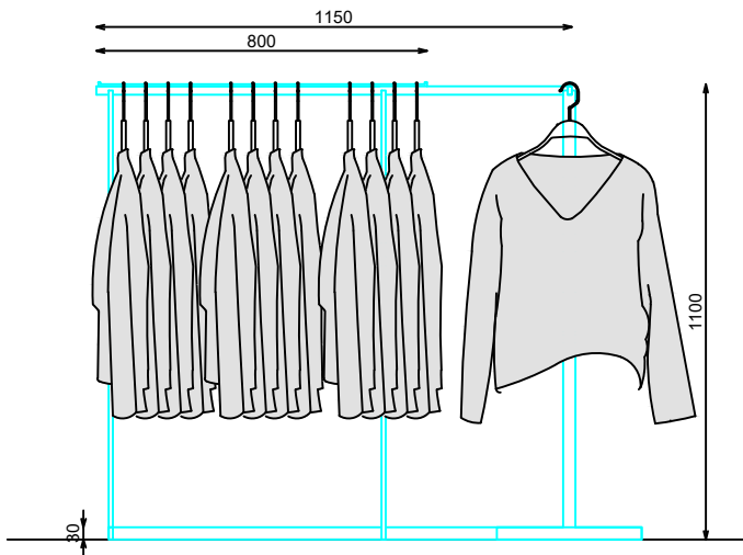
ALZADO LATERAL
