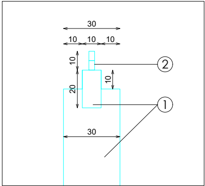
DETALLE A
