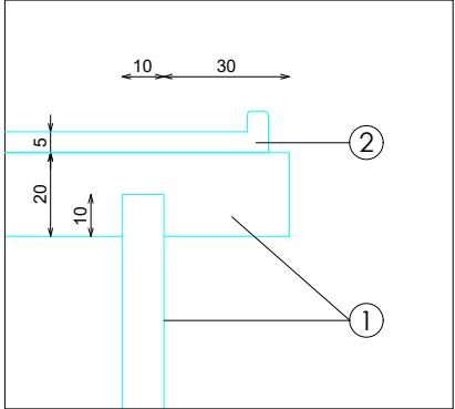
DETALLE B
