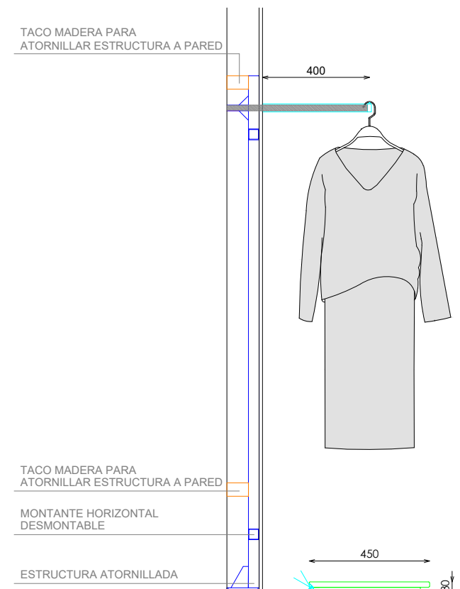
SECCION
