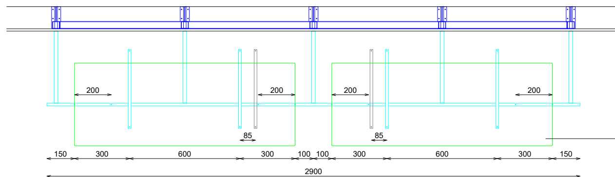
PLANTA
