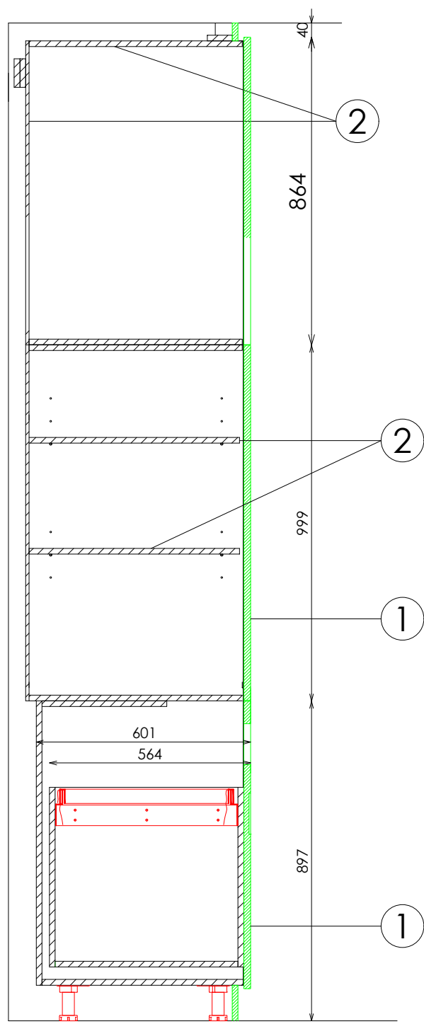
SECCIÓN MOVERAS
