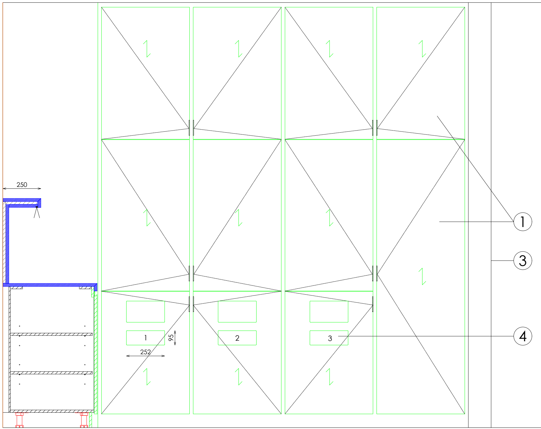
ALZADO EXTERIOR
