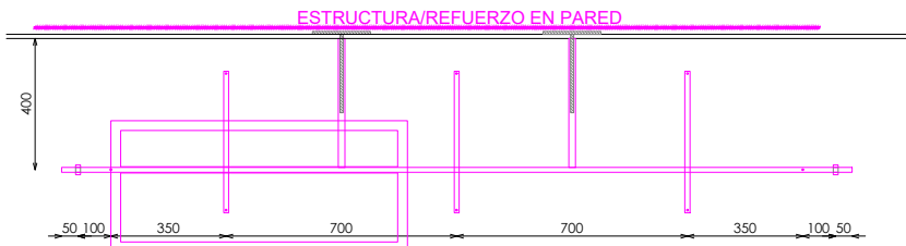
PLANTA
