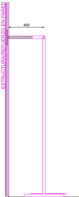
SECCION
