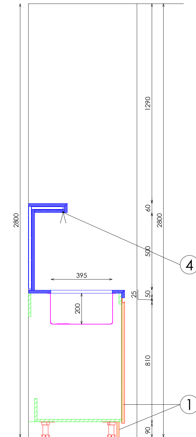
SECCIÓN MODULO FREGADERO
