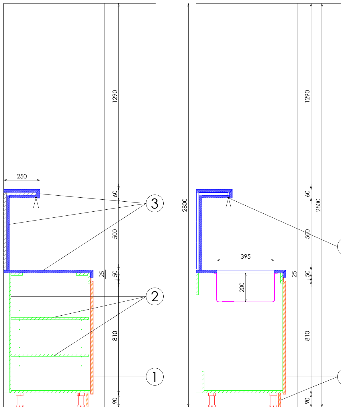
SECCIÓN MODULOS
