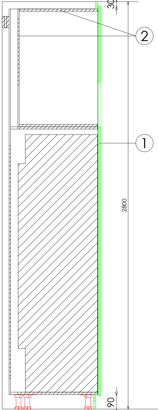
SECCIÓN NEVERA
