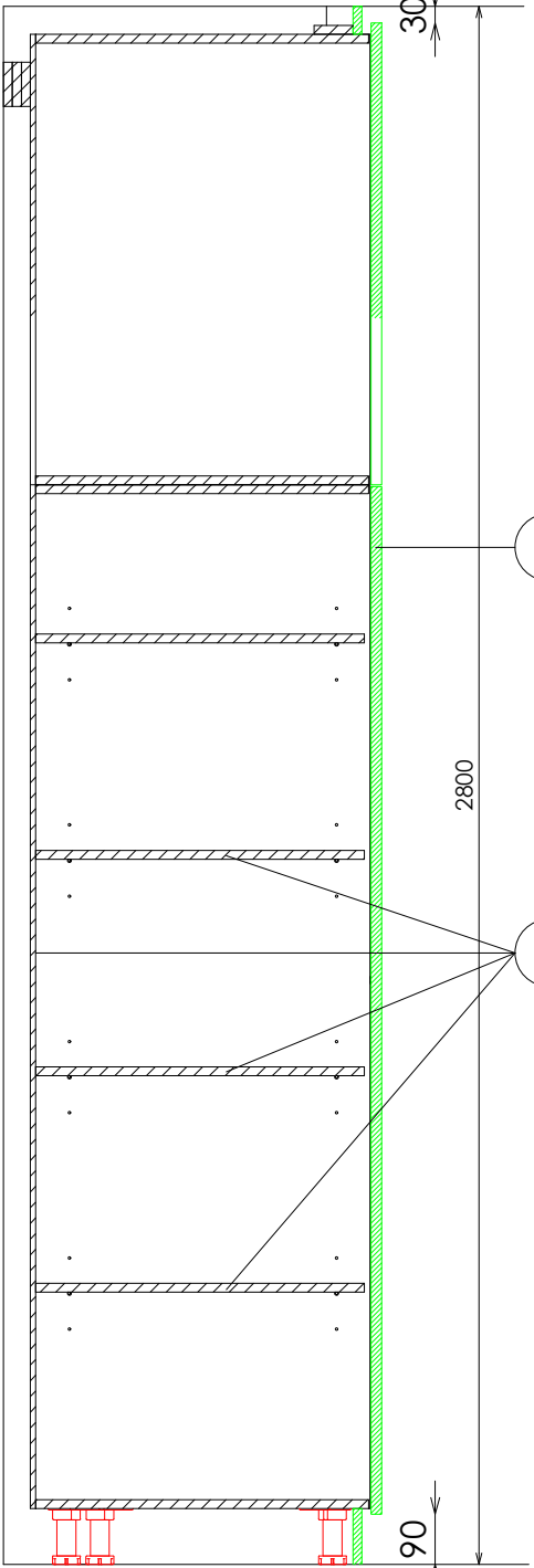
SECCIÓN ALMACENAJE
