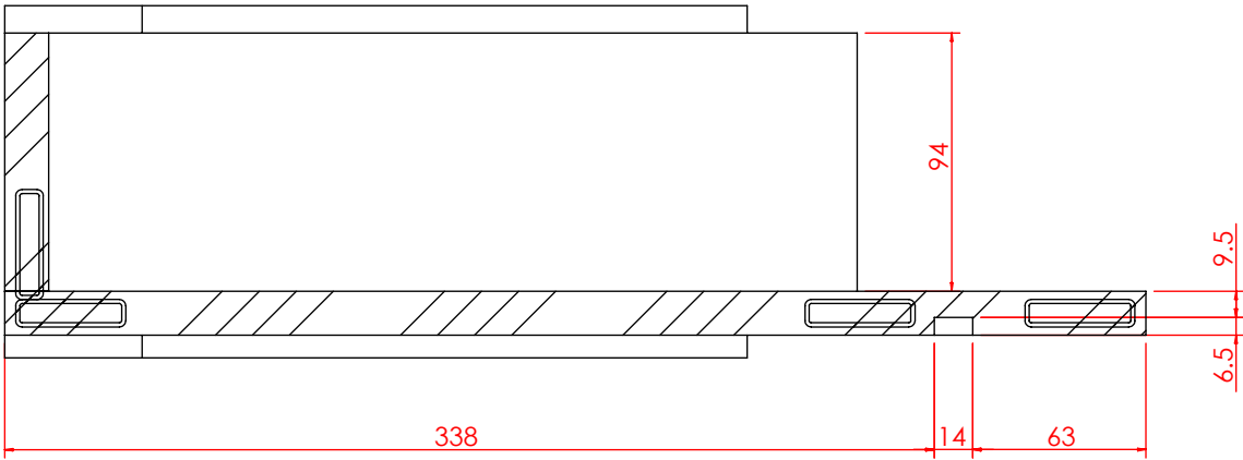
局部视图 AI 比例 1 : 3
