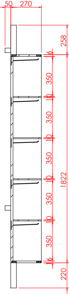
剖面 AH-AH
