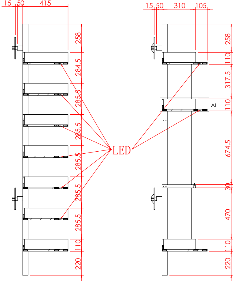
剖面 AK-AK
