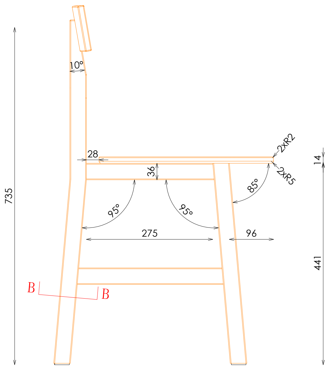
ALZADO LATERAL
