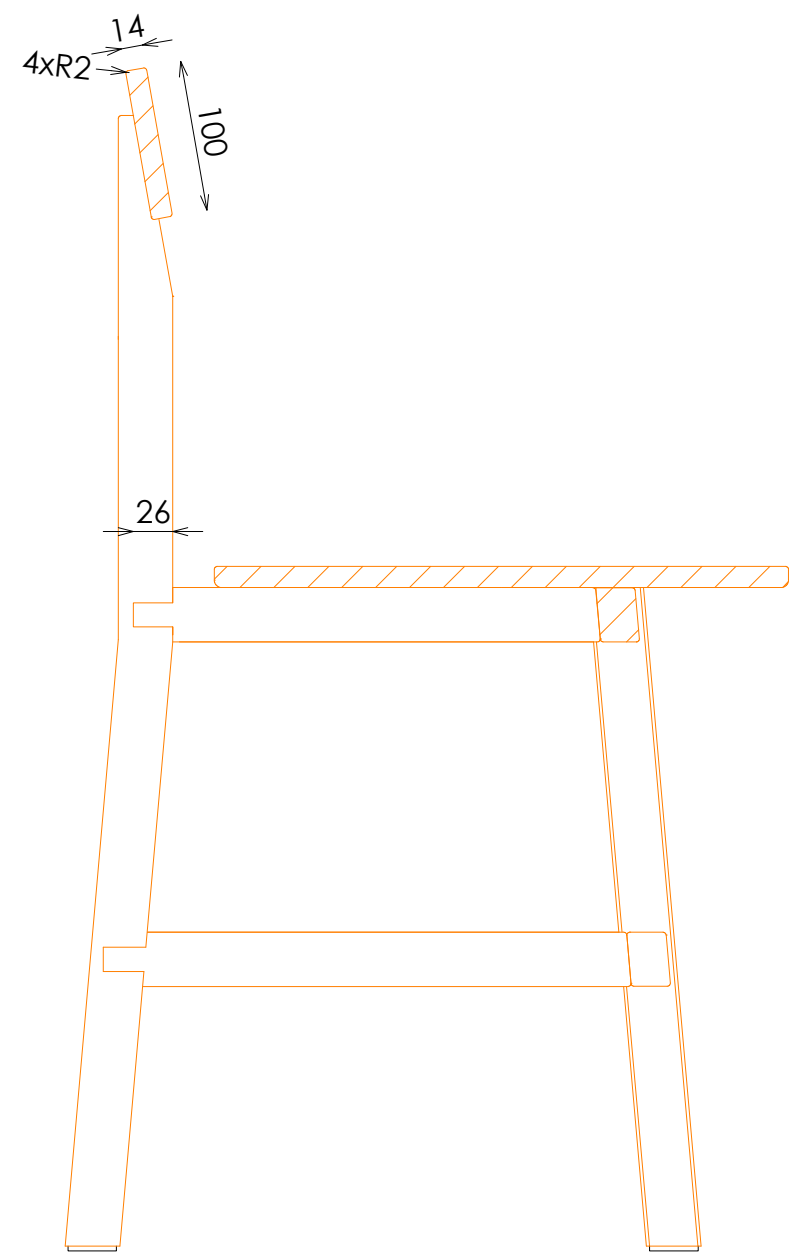
SECCION C-C
