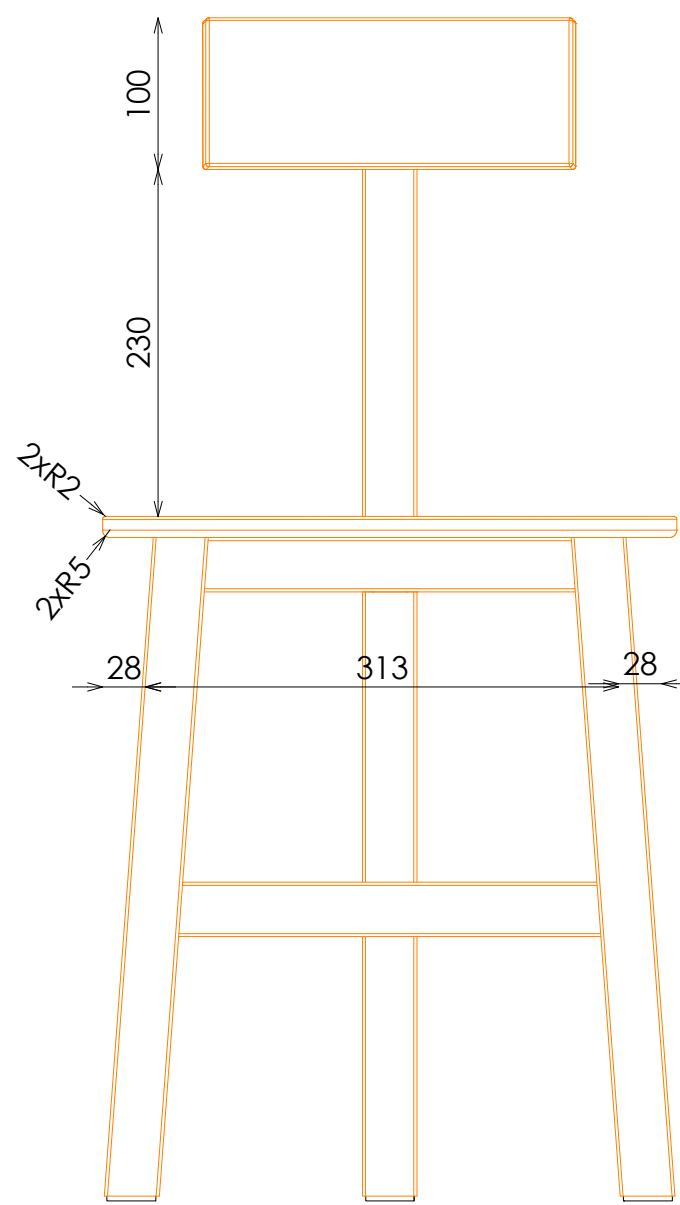
ALZADO FRONTAL
