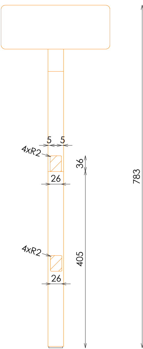
SECCIÓN A-A
