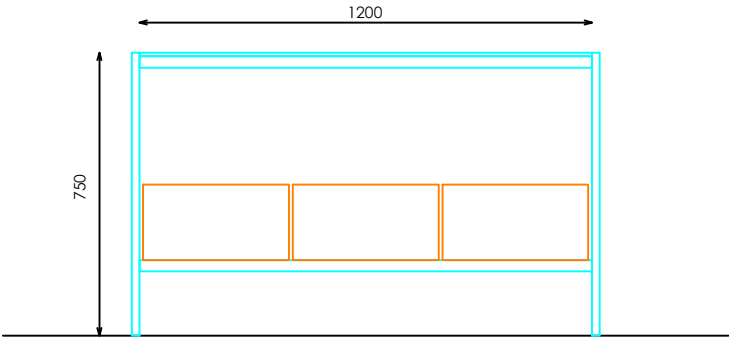
ALZADO LATERAL
