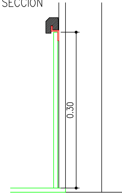
SECCIÓN
