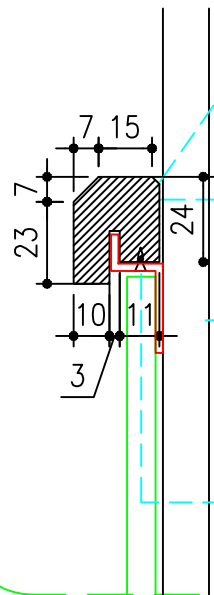
DETALLE MOLDURA
