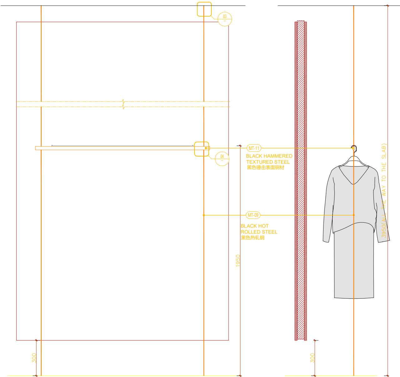
2 正立面 1:10 FRONT ELEVATION
