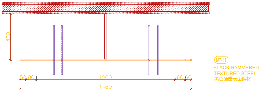
1 平面图 1:10 PLAN
