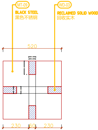
1 平面图 1:10 PLAN
