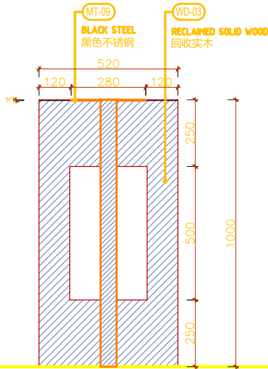
6 侧立面 1:10 SIDE ELEVATION
