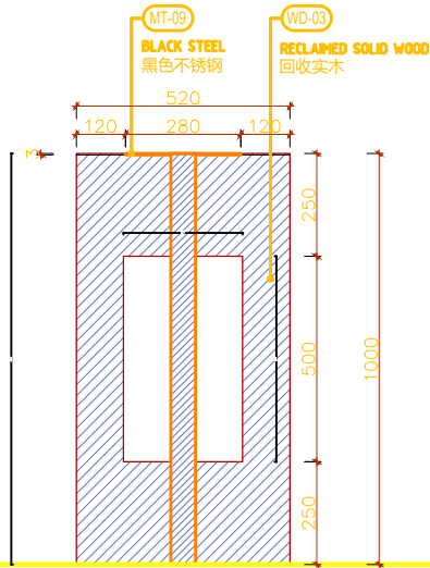
2 正立面 1:10 FRONT ELEVATION
