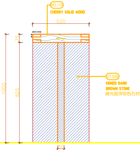
2 正立面 1:10 FRONT ELEVATION
