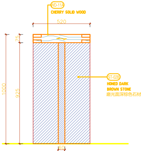
6 侧立面 1:10 SIDE ELEVATION
