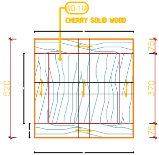
1 平面图 1:10 PLAN
