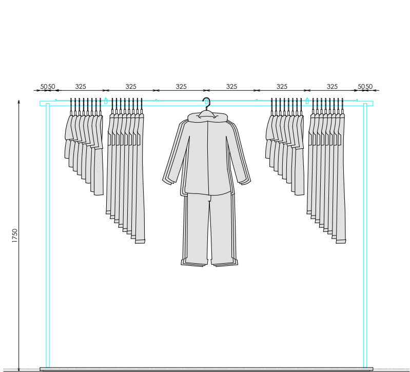
ALZADO FRONTAL
