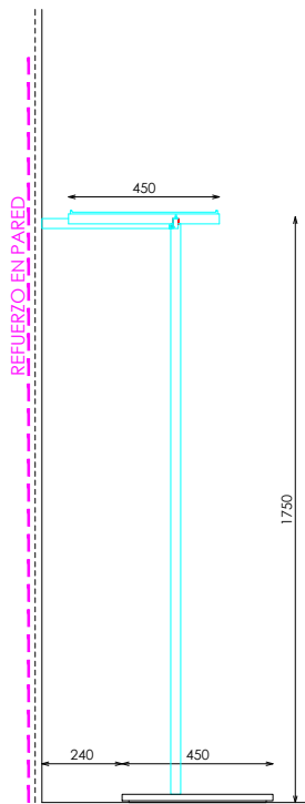
PERFIL
