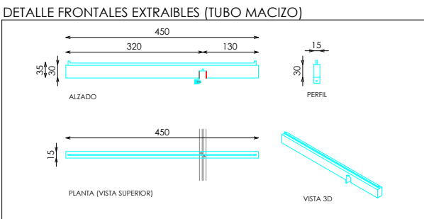
DETALLE FRONTALES EXTRAIBLES (TUBO MACIZO)
