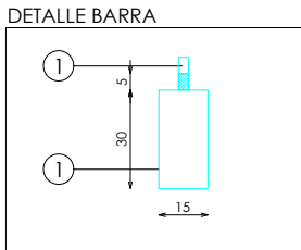
DETALLE BARRA
