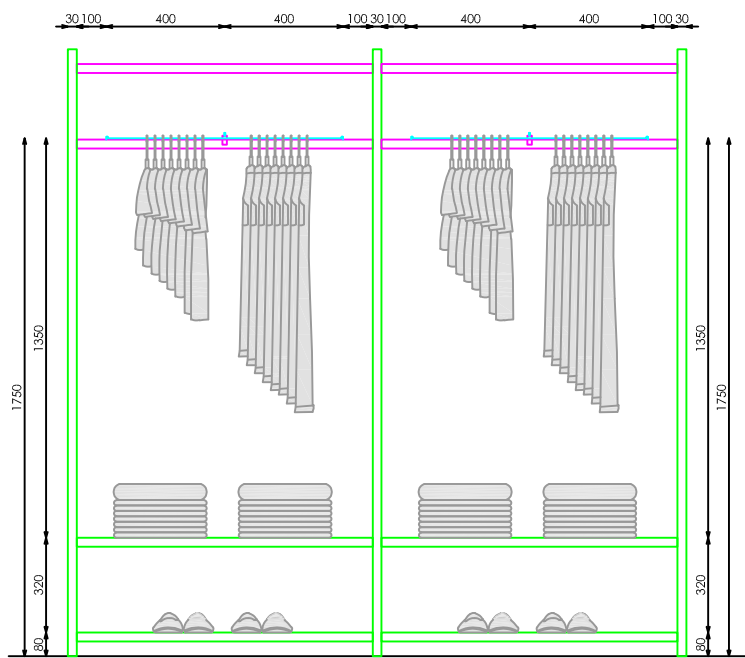
ALZADO
