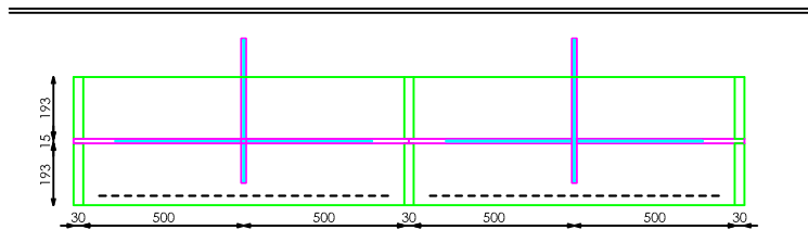
PLANTA
