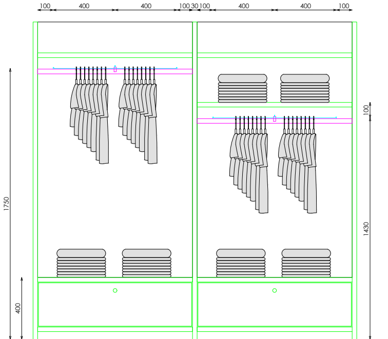
ALZADO
