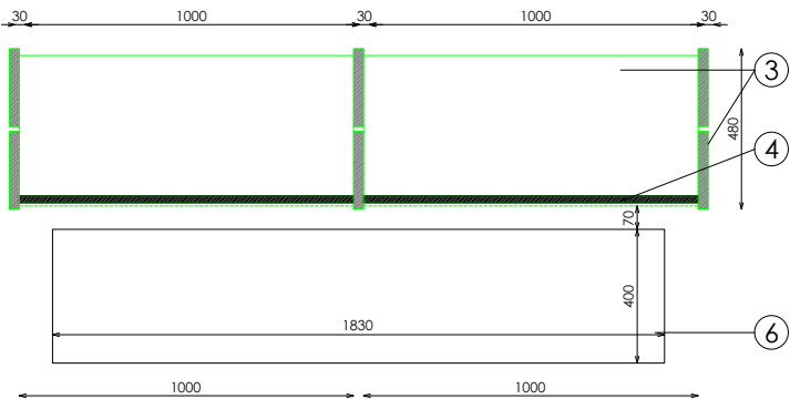
PLANTA (TARIMA)
