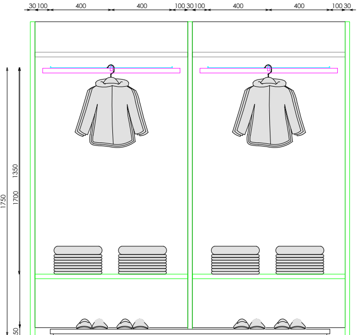
ALZADO
