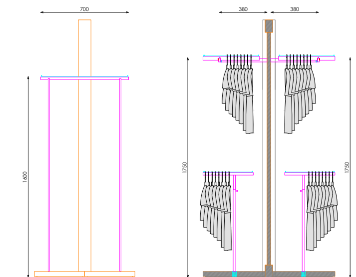
PERFIL DERECHO
