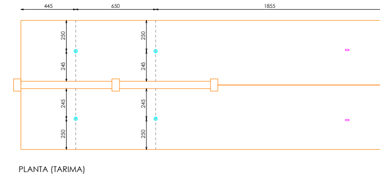
PLANTA (TARIMA)
