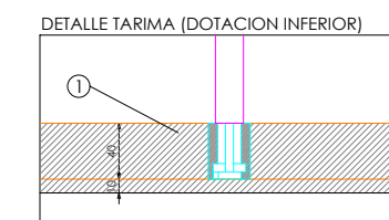
TAPON EXTRAIBLE TARIMA
