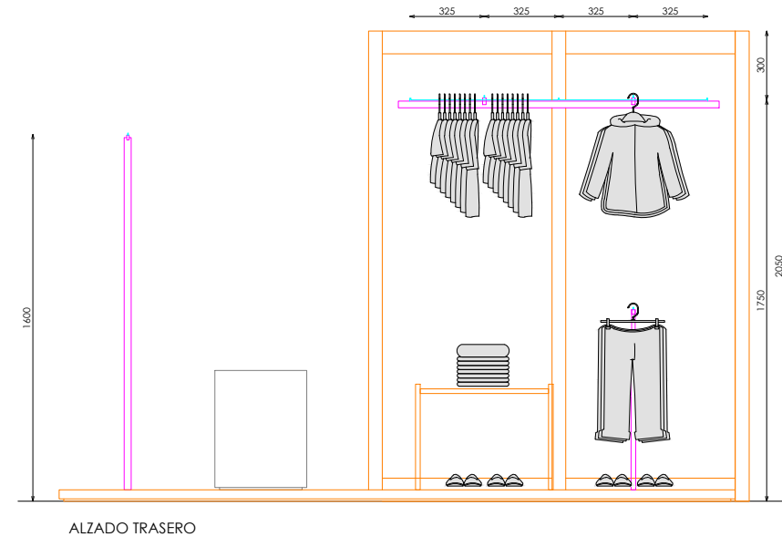
ALZADO TRASERO
