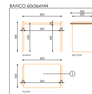
BANCO 60x36xH44
