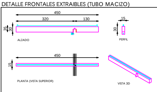
DETALLE FRONTALES EXTRAIBLES (TUBO MACIZO)
