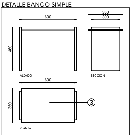
DETALLE BANCO SIMPLE
