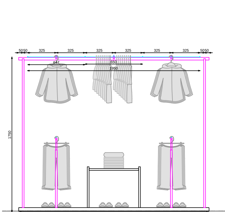
ALZADO FRONTAL
