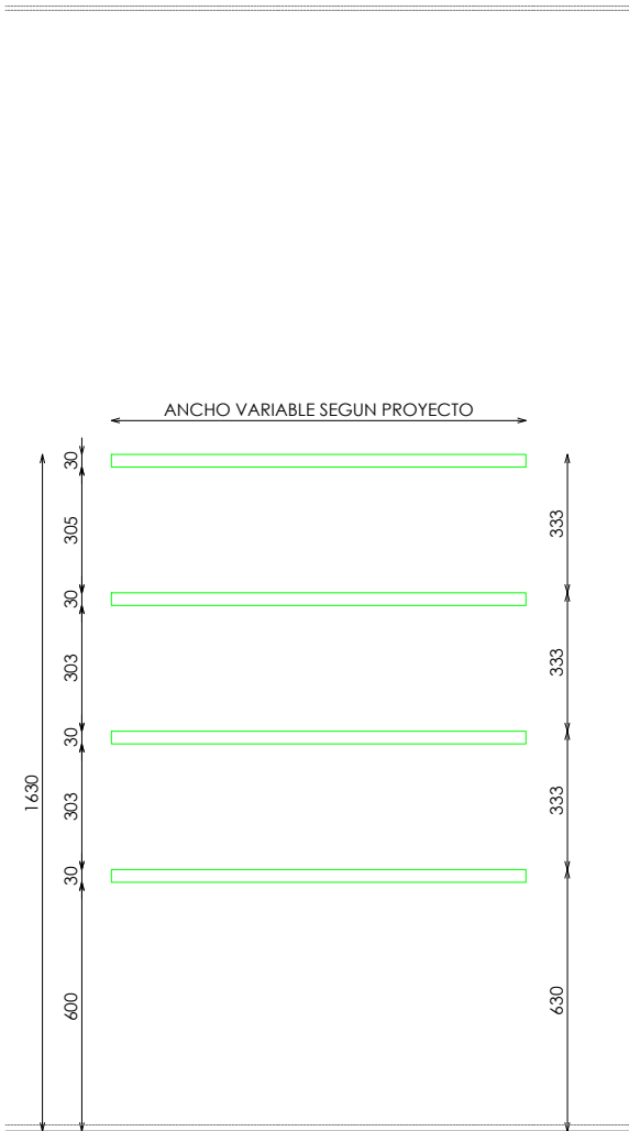
ALZADO
