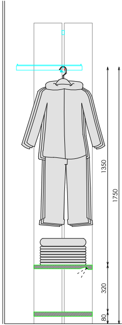
SECCION
