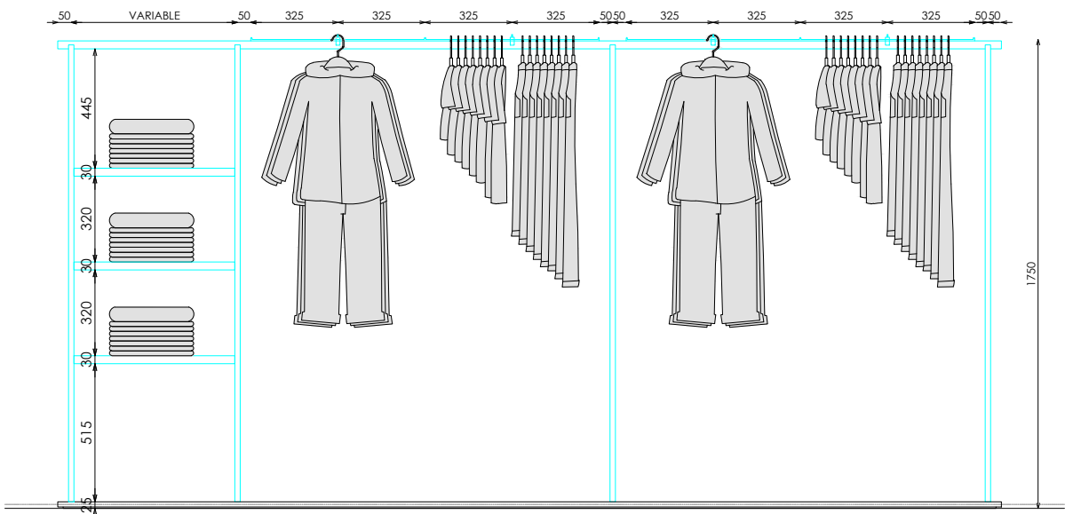
ALZADO FRONTAL
