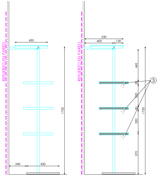
PERFIL
