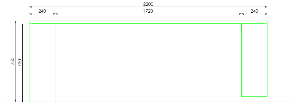
ALZADO
