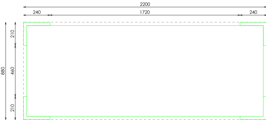
PLANTA (PATAS)
