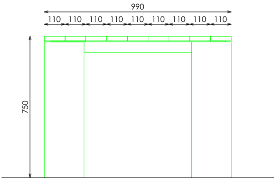
PERFIL
