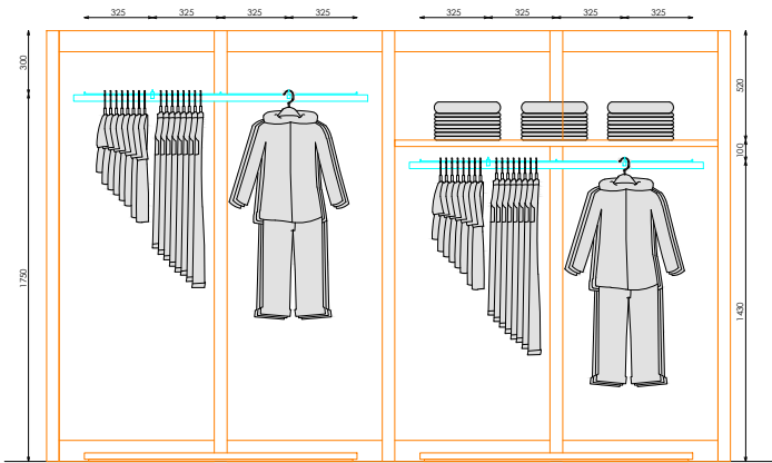
ALZADO TRASERO
