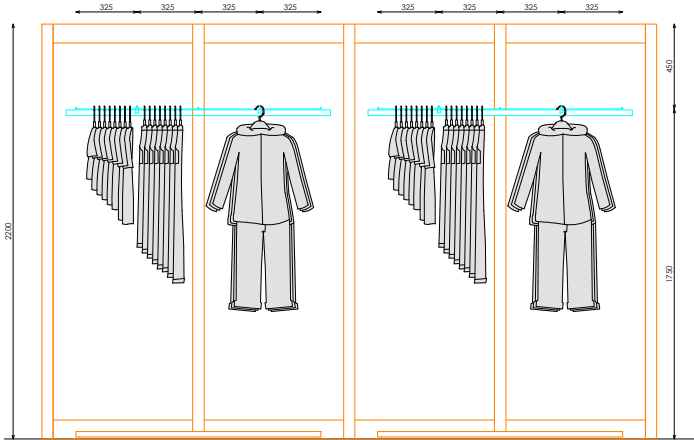
ALZADO FRONTAL
