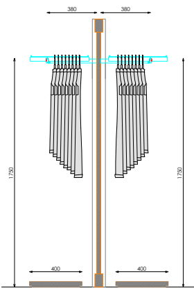
SECCION
