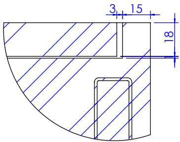
局部视图 AH 比例 1 : 2
