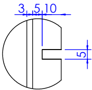
局部视图 AI 比例 1 : 2
