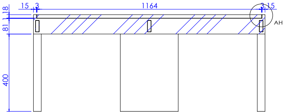
剖面 AG-AG
