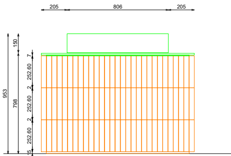
PERFIL
