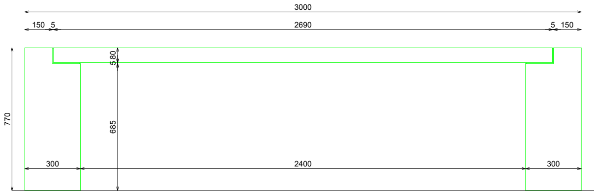
ALZADO
