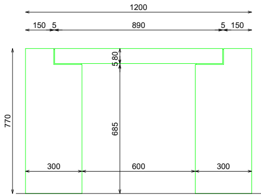
PERFIL
