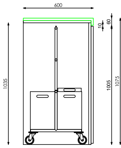
SECCION
