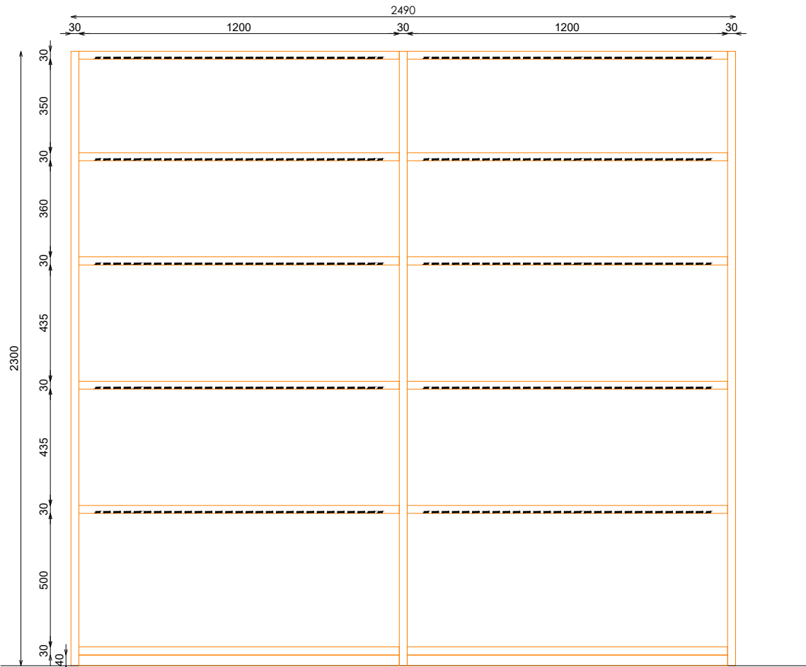
ALZADO
