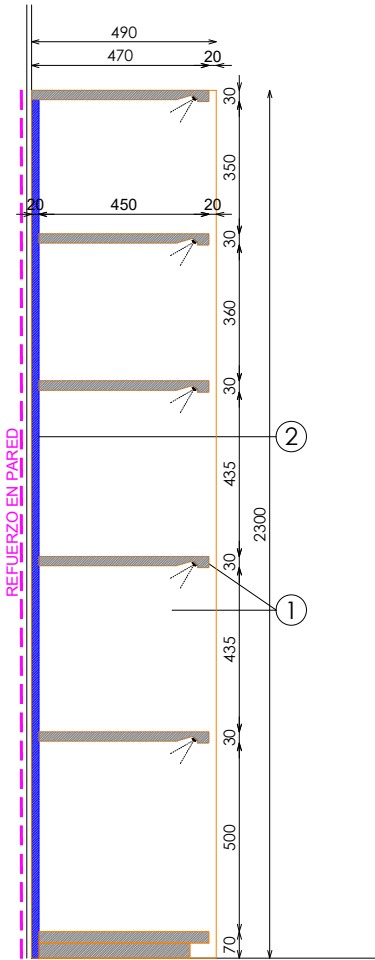
SECCION
