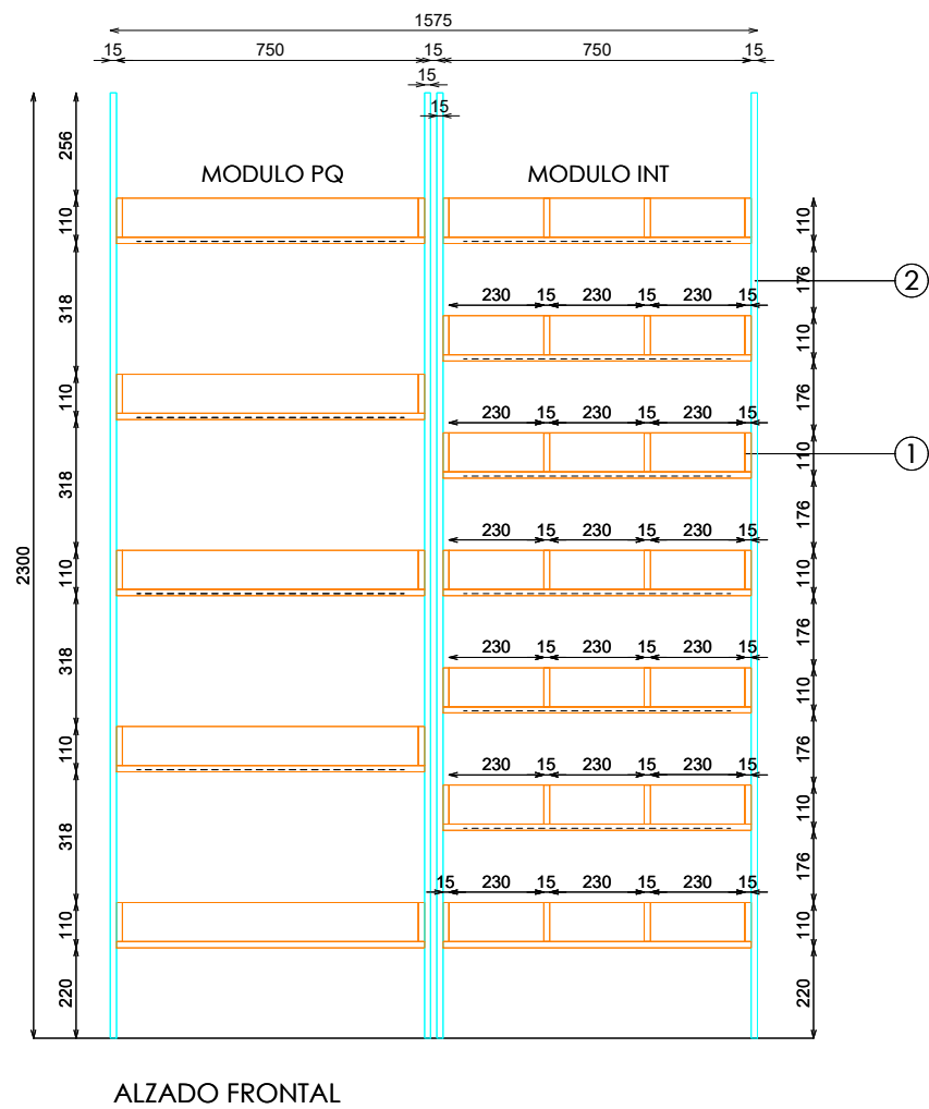
ALZADO FRONTAL
