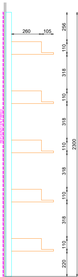
PERFIL MODULO PQ
