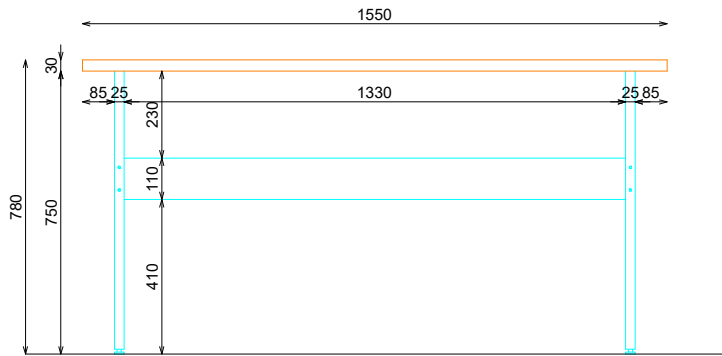
ALZADO FRONTAL
