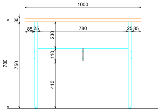
ALZADO LATERAL
