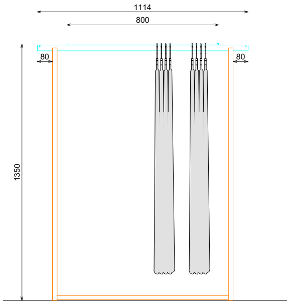
ALZADO
