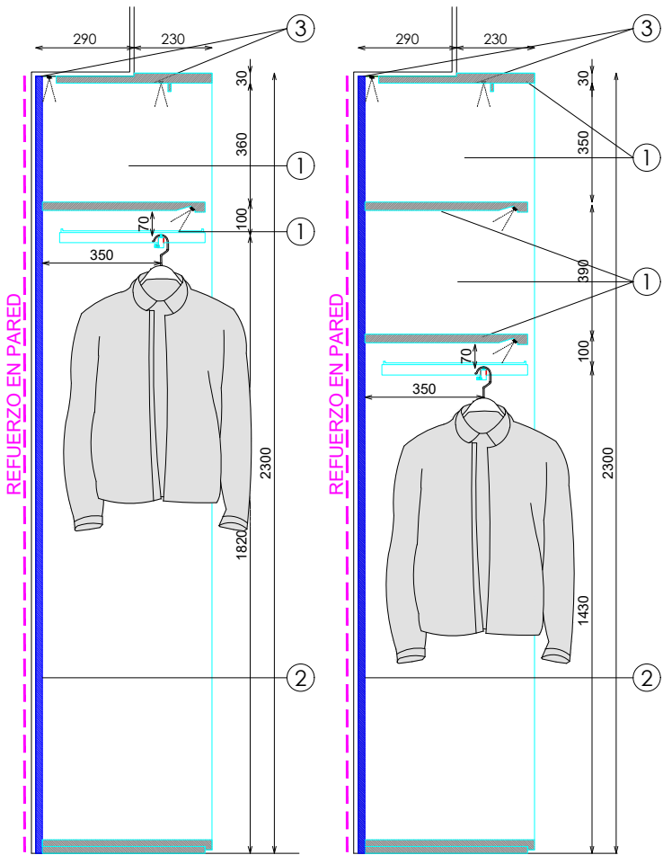
SECCION BARRA ALTA
