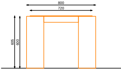
ALZADO FRONTAL
