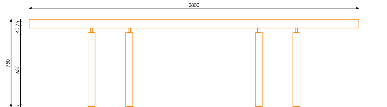
ALZADO LATERAL
