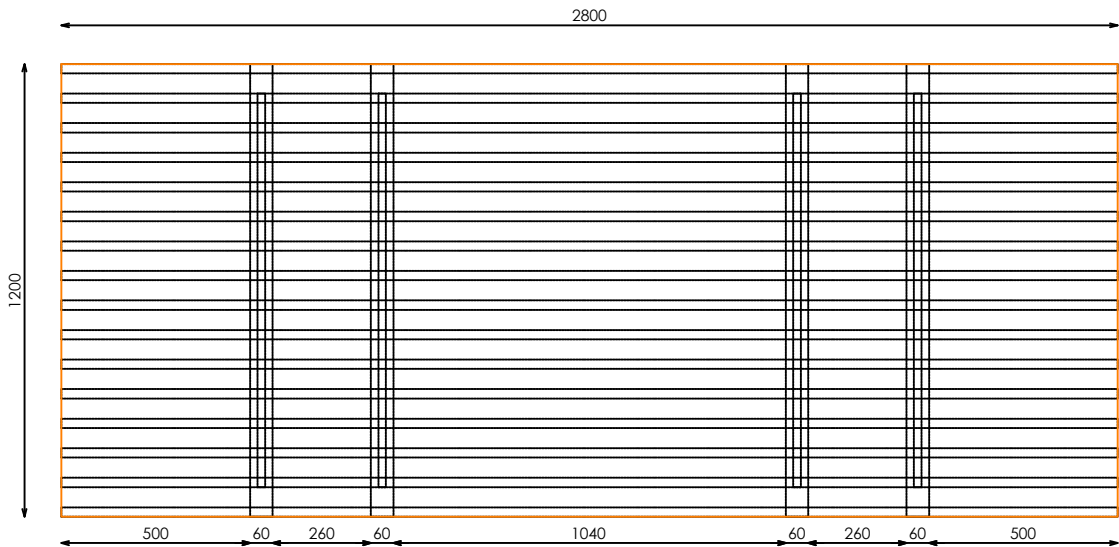
PLANTA
