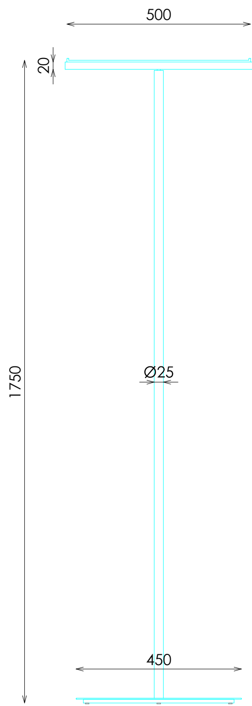
ALZADO
