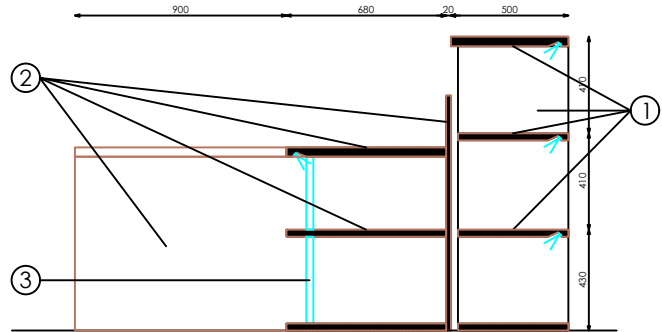
SECCIÓN
