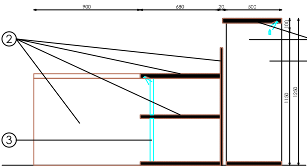
SECCIÓN
