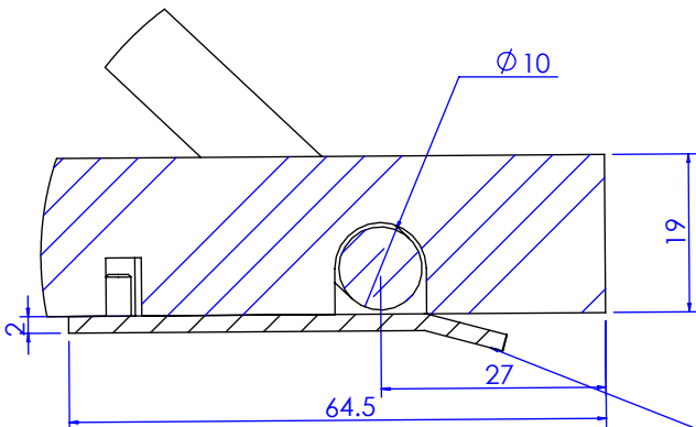
局部视图 B 比例 1 : 1
