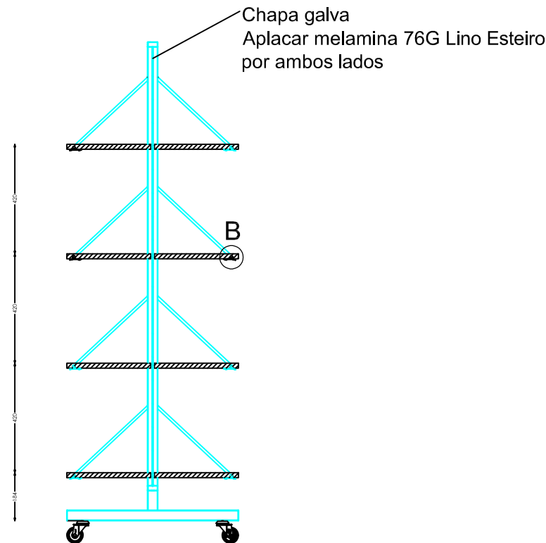
SECCIÓN A-A
