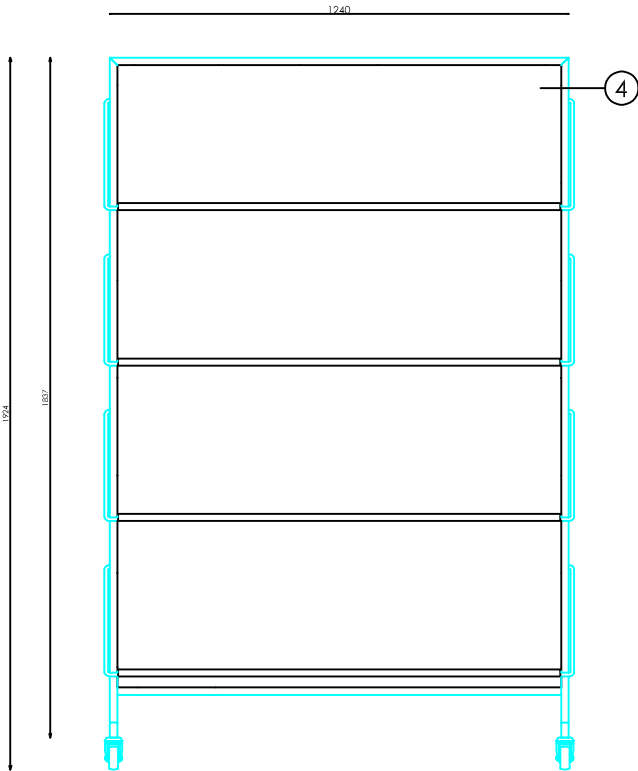
ALZADO FRONTAL
