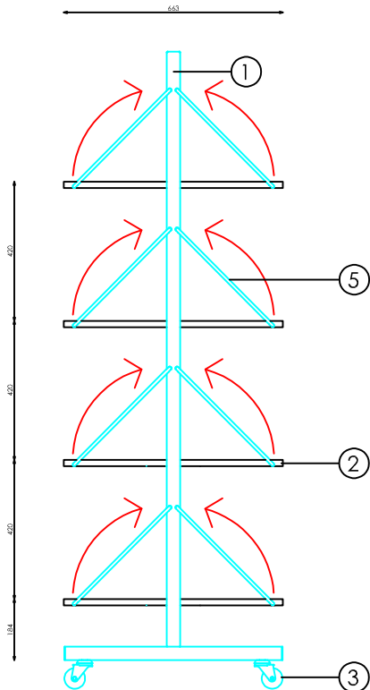
ALZADO LATERAL
