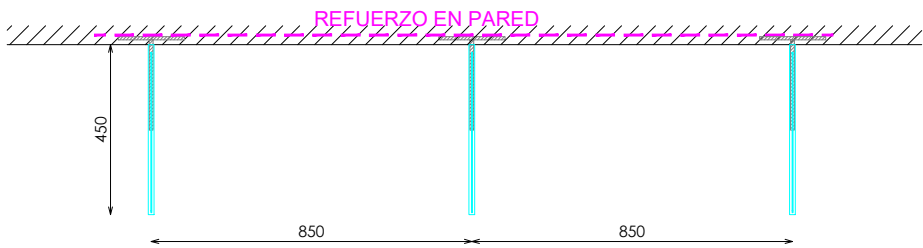
PLANTA
