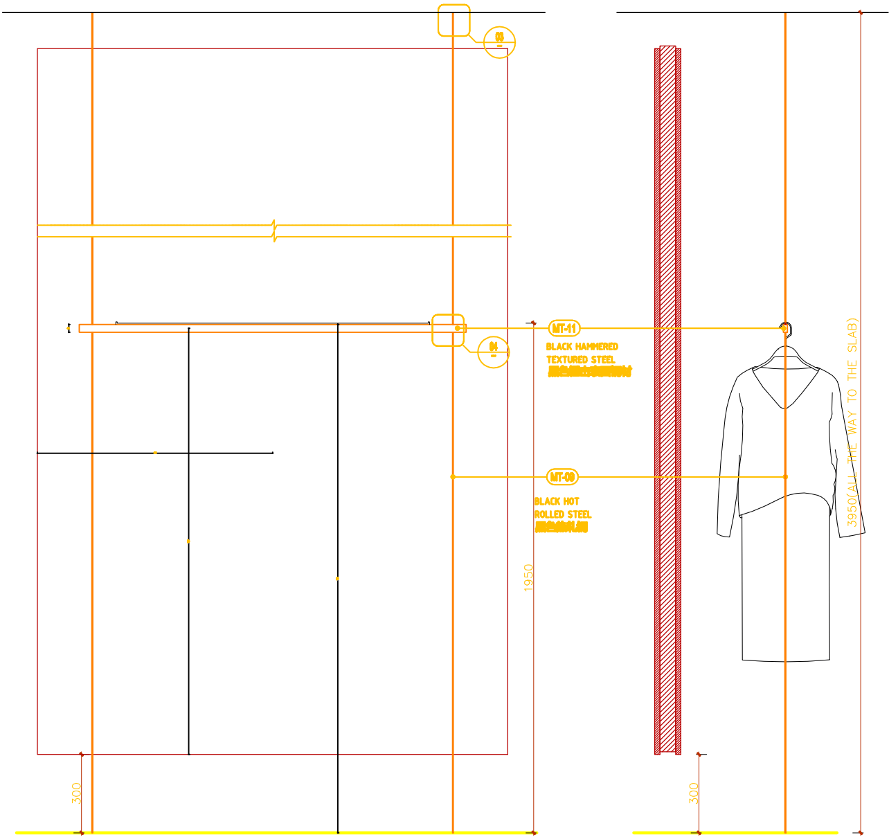
2 1:10 正立面 FRONT ELEVATION
