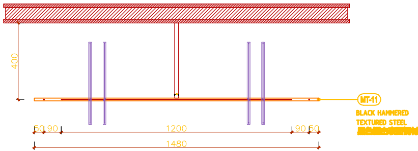
1 1:10 平面图 PLAN
