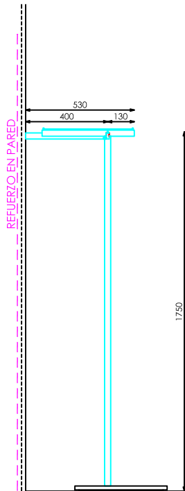
SECCION
