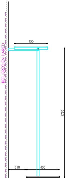
PERFIL
