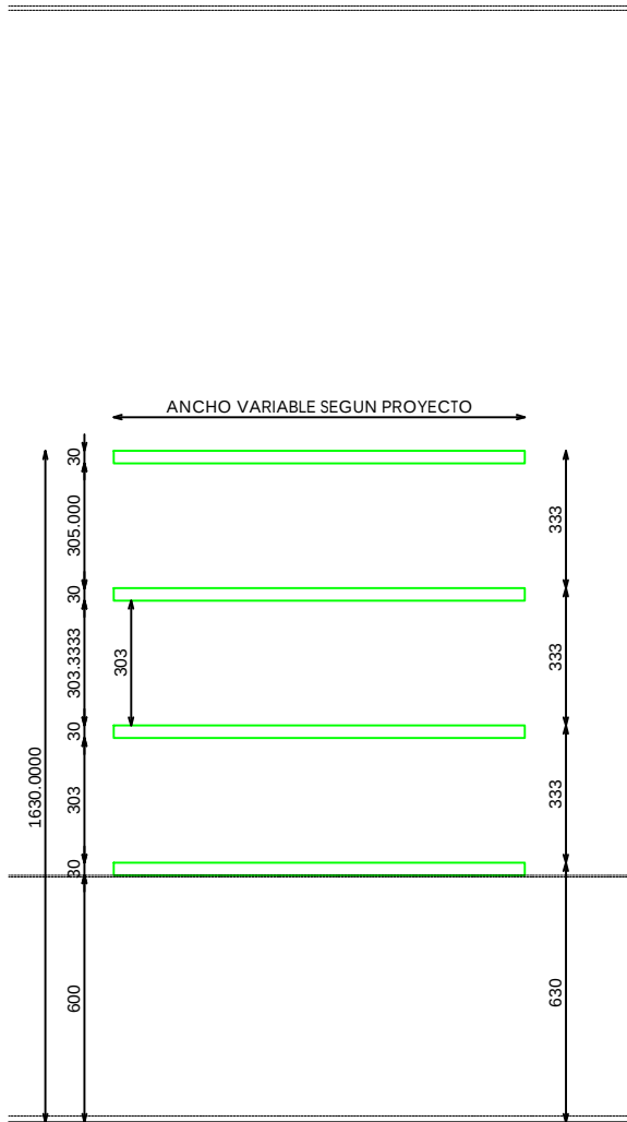
ALZADO
