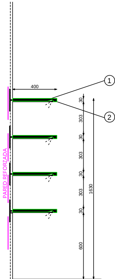
PERFIL
