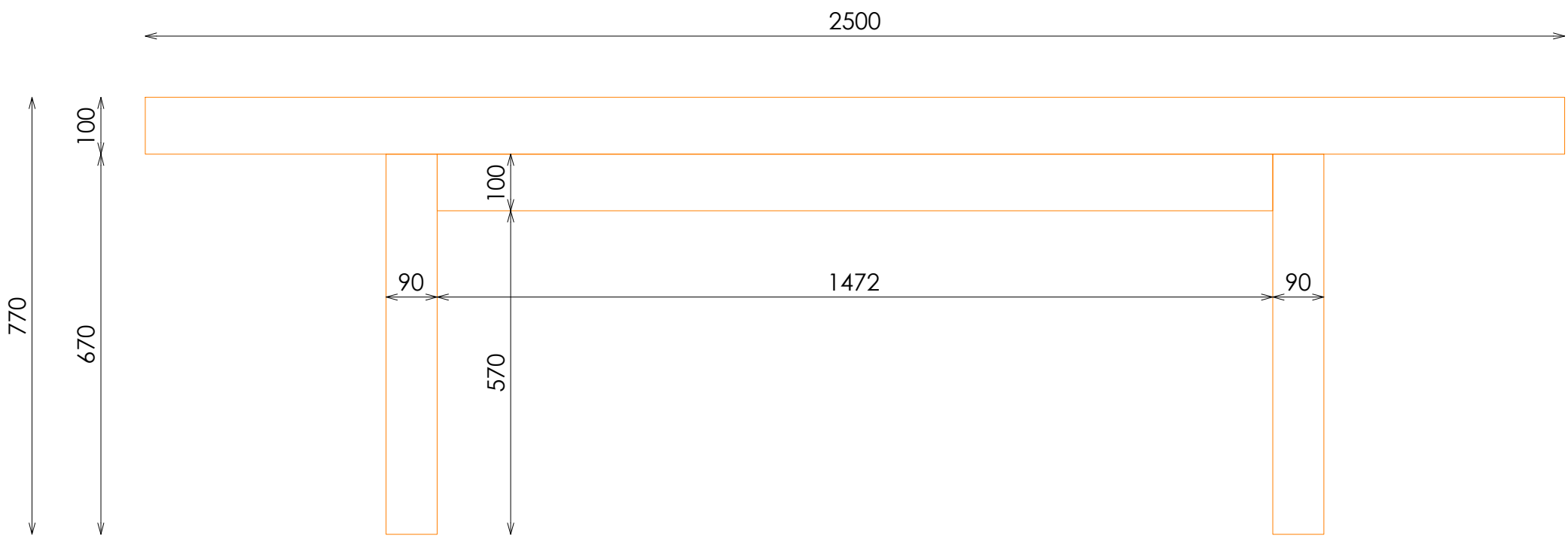
ALZADO FRONTAL
