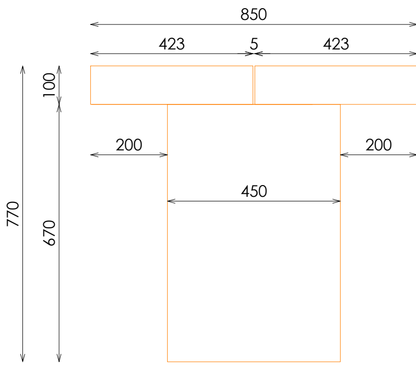
ALZADO LATERAL
