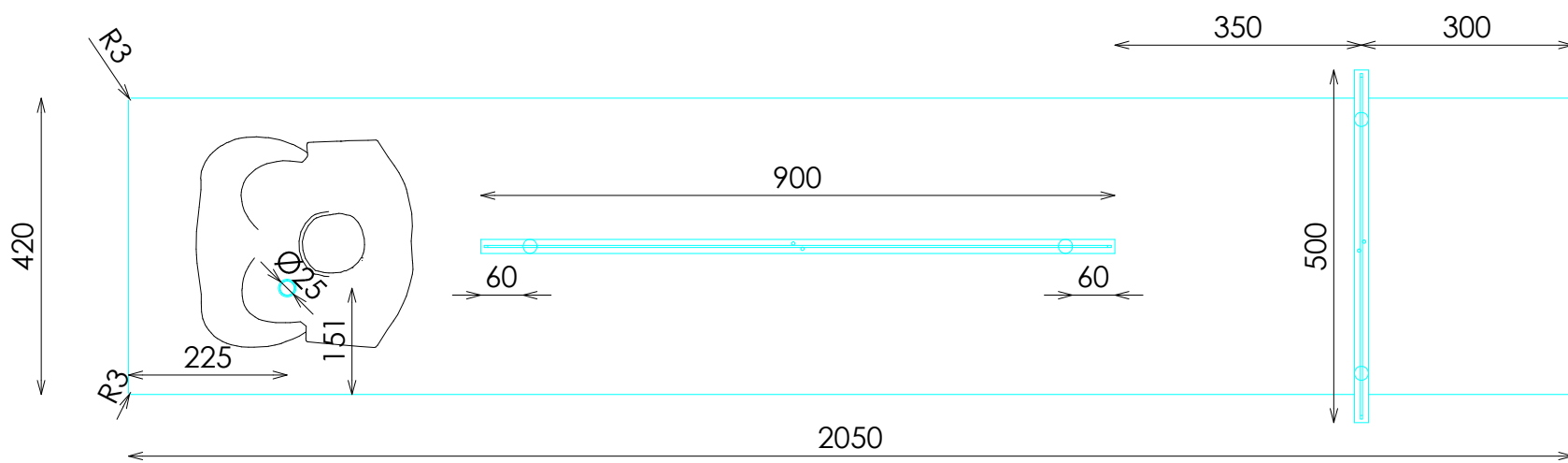
ALZADO LATERAL
