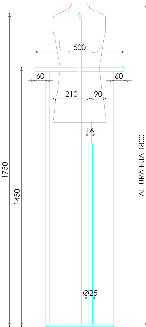
ALZADO FRONTAL
