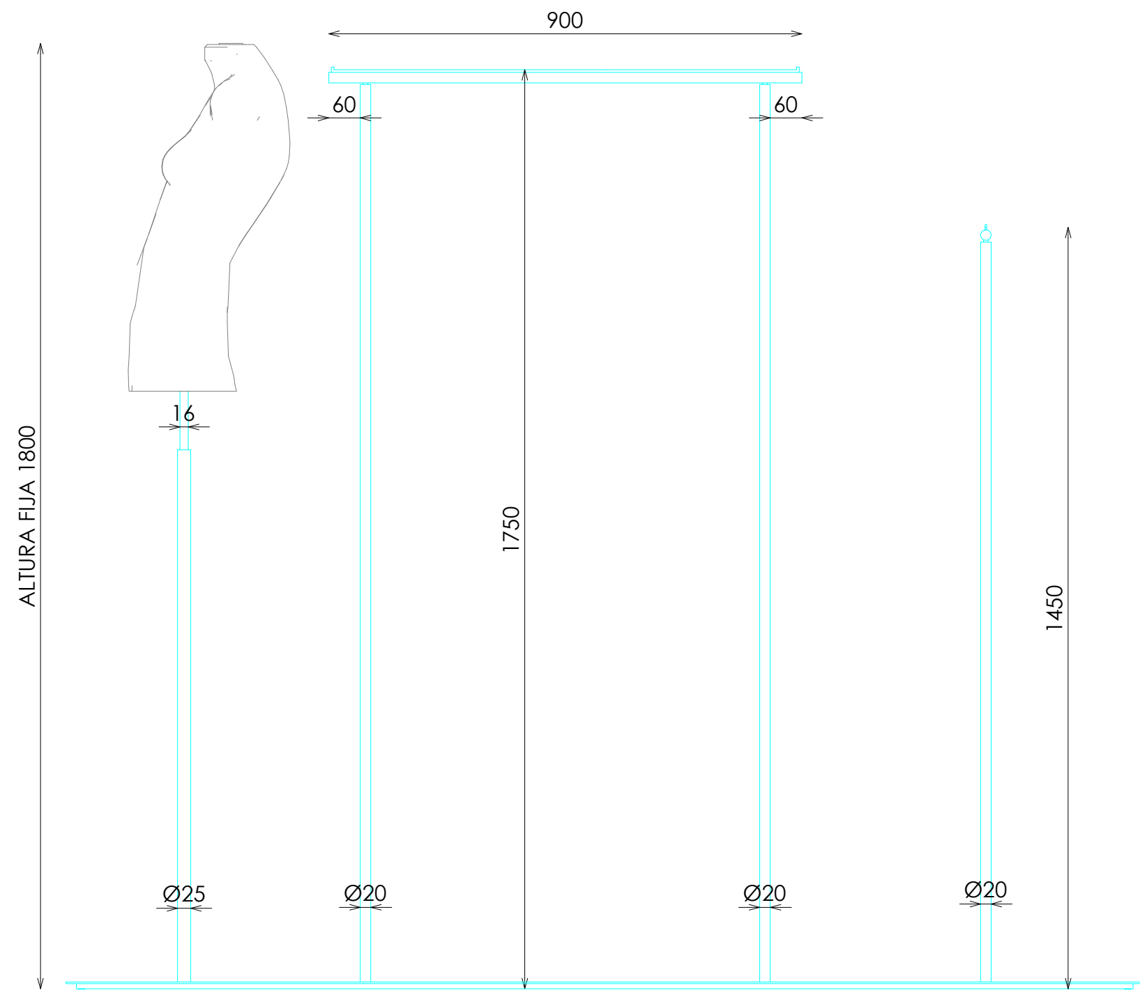
ALZADO LATERAL
